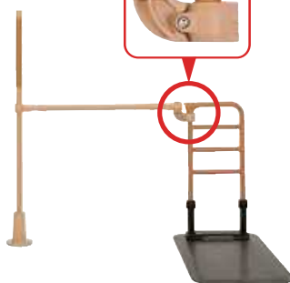
垂直型手すり【バディーI】と連結
